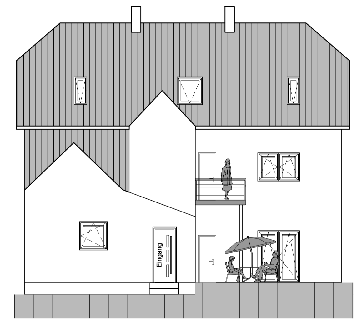
GARTENANSICHT
