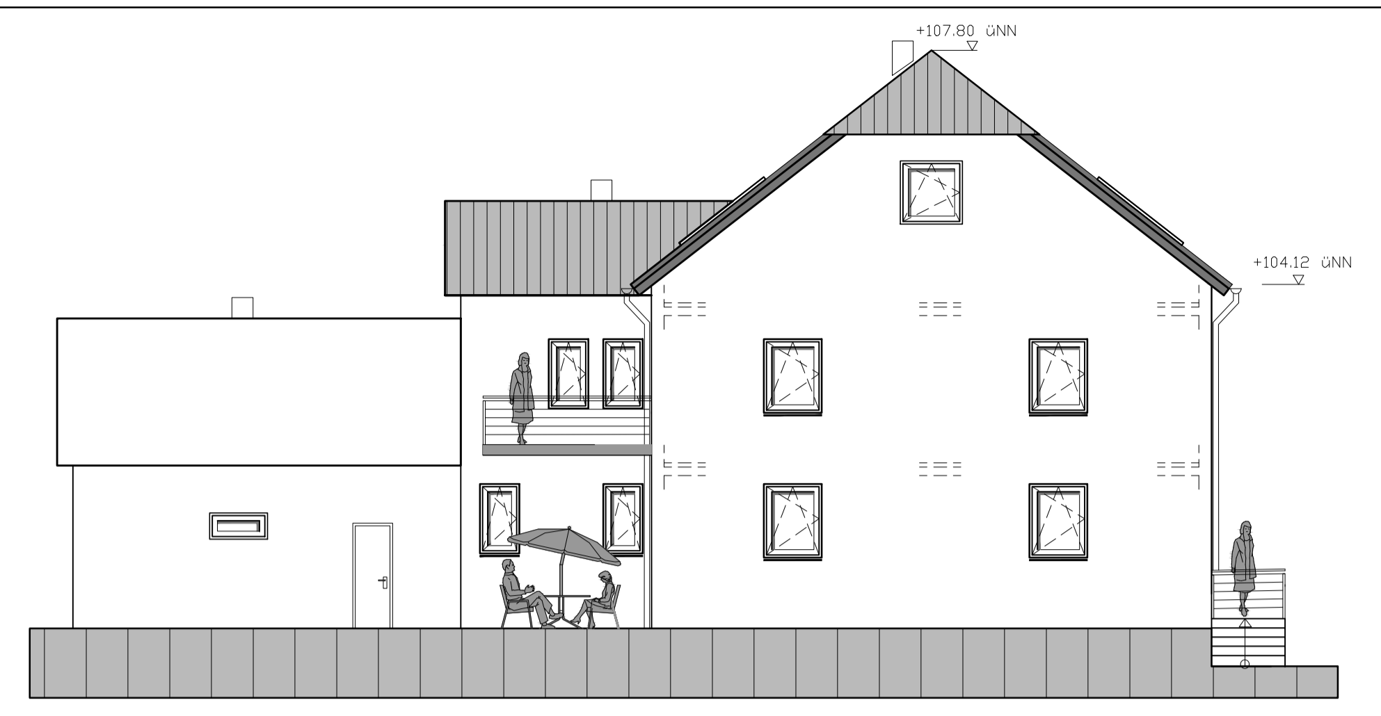
2.GIEBELANSICHT
