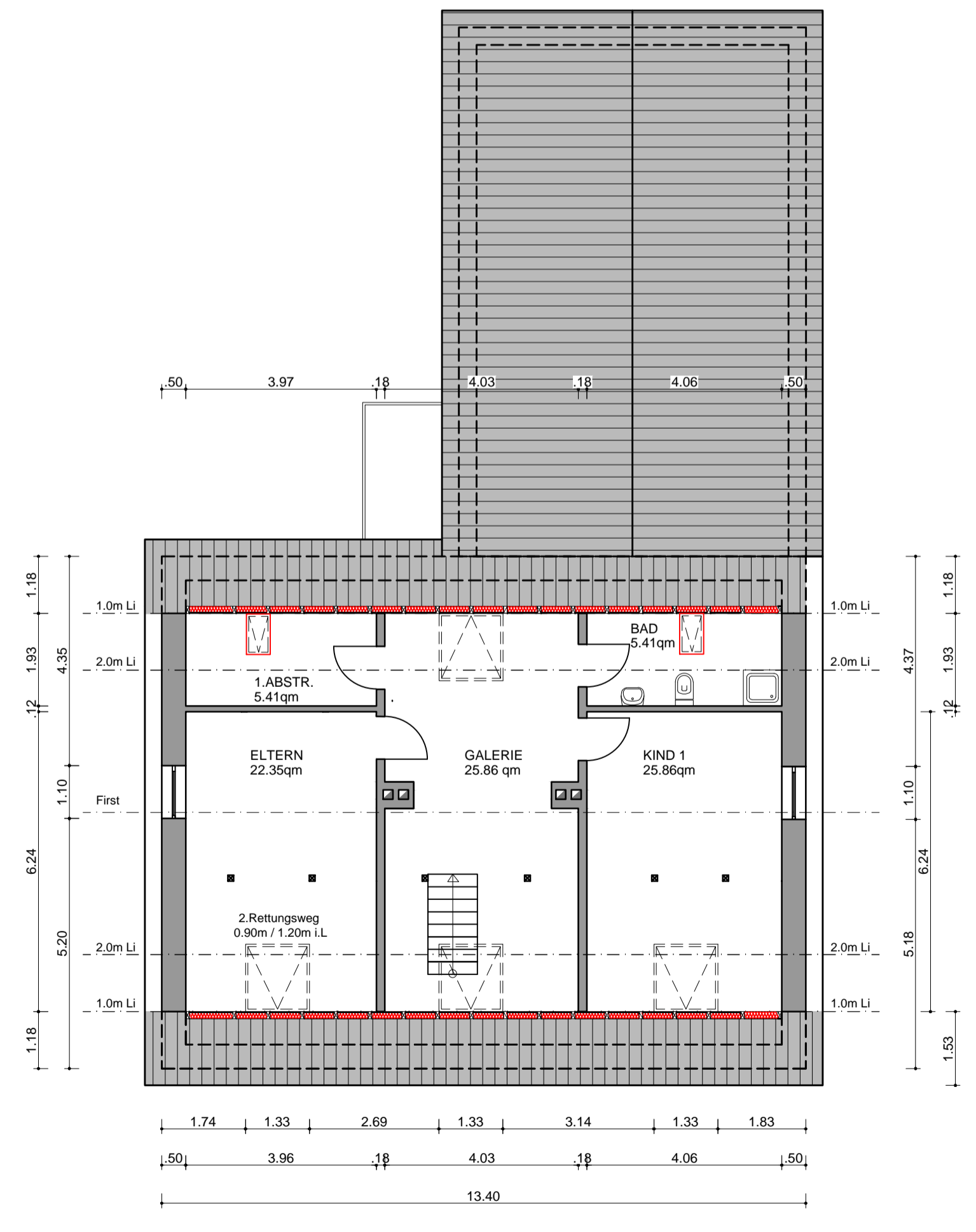
DACHGESCHOSS
