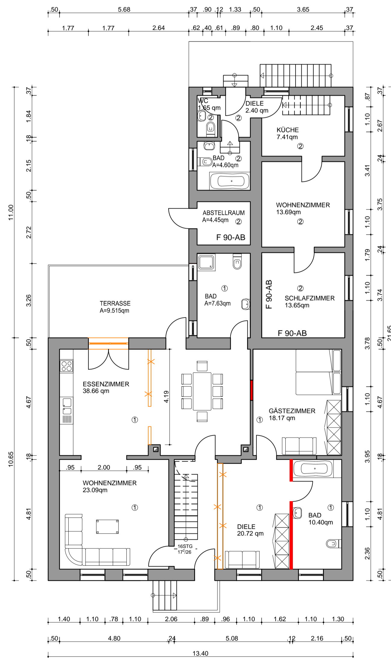
ERDGESCHOSS
